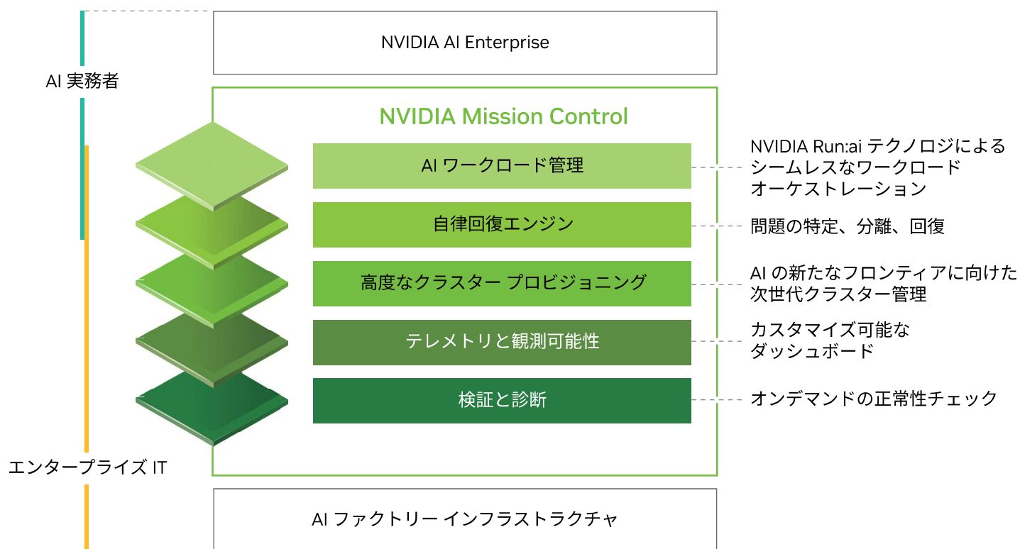
NVIDIA DGX ソフトウェア スタック
